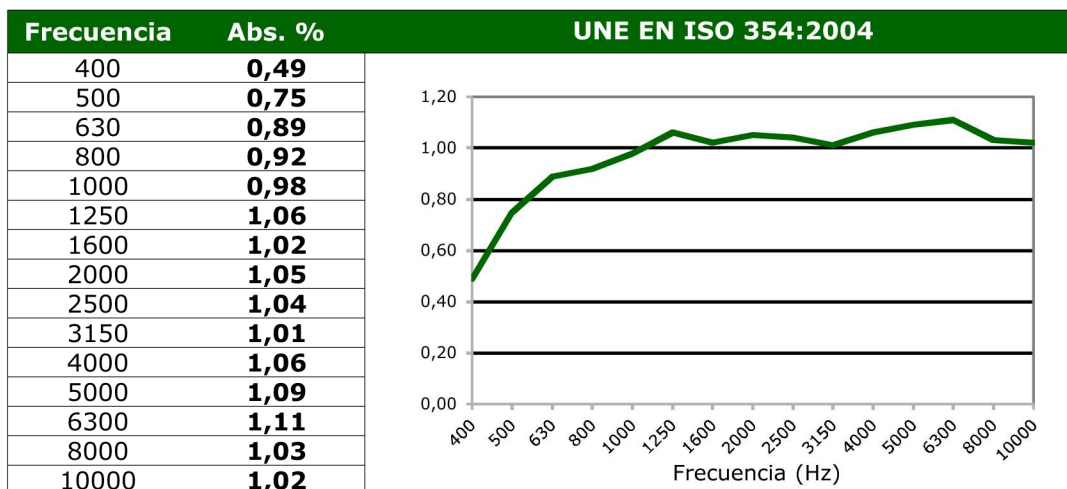
Absorció acústica en cabina alpha
