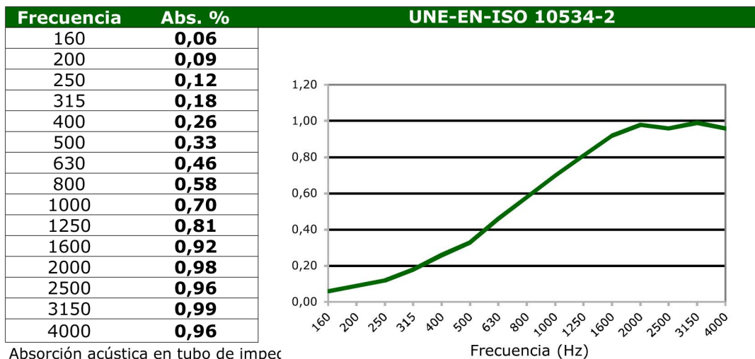
Absorció acústica en tubo de impec
