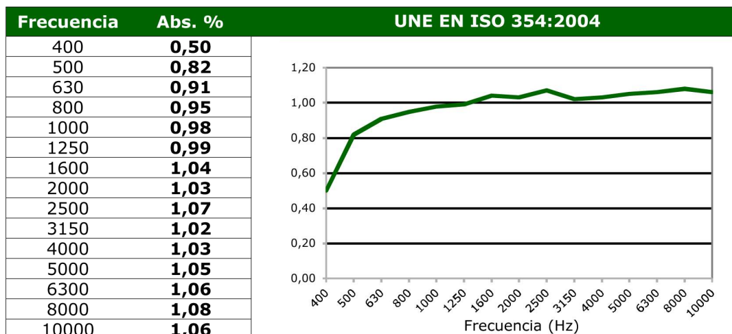
Absorción acústica en cabina alpha
